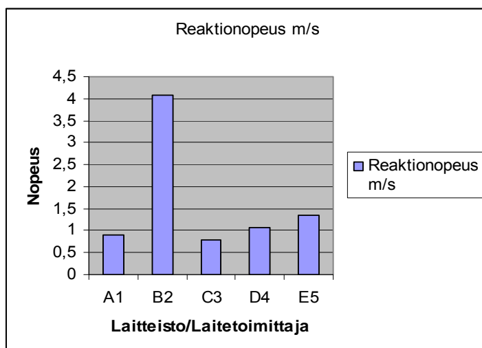
Kuvio 2. Puolivälitestauksen ajat m/s putken tai kapillaariputken päästä keskukseen
