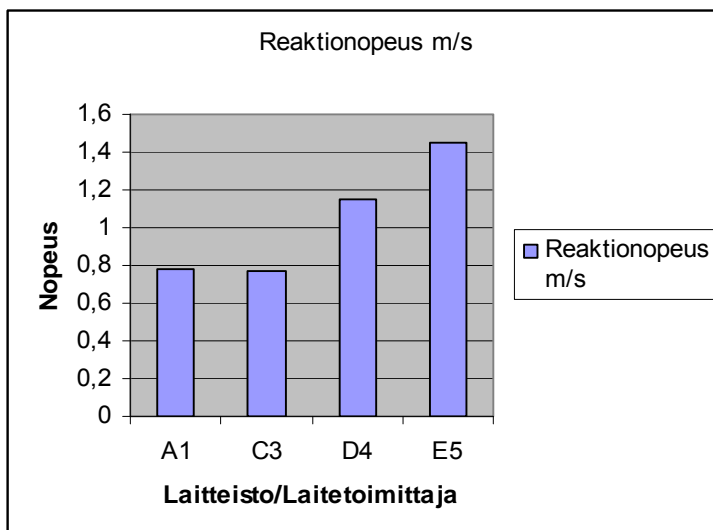
Kuvio 1. Alkutestien ajat m/s, putken päästä palovaroitinkeskukselle
